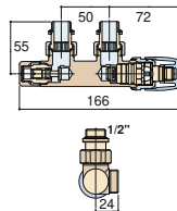
ПРАВЫЙ ПРЯМОУГОЛЬНЫЙ ВЕНТИЛЬ KRISTAL, МЕЖСЕБЕВОЕ РАССТОЯНИЕ МЕЖДУ ТРУБАМИ 50 ММ, С ТЕРМОСТАТОМ - МАТОВАЯ ОТДЕЛКА KRISTAL VALVE SQUARE RIGHT PIPE CENTRES 50 MM WITH THERMOSTATIC OPTION - SATIN FINISHING
