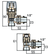
ПРЯМОУГОЛЬНЫЙ ВЕНТИЛЬ KRISTAL С ТЕРМОСТАТОМ, ХРОМИРОВАННЫЙ KRISTAL VALVE SQUARE WITH THERMOSTATIC OPTION CHROMED FINISHING
