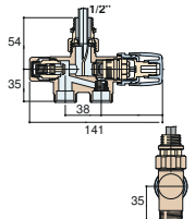
ДВУНАПРАВЛЕННЫЙ ВЕНТИЛЬ KRISTAL С НИЖНИМ ВПУСКОМ, РАСПОЛОЖЕННЫМ СПРАВА, И ТЕРМОСТАТОМ - БЕЛЫЙ R01 - RAL 9010 VALVE KRISTAL BIDIRECTIONAL UNDERNEATH INLET AT RIGHT SIDE WITH THERMOSTATIC OPTION - WHITE R01 - RAL 9010
