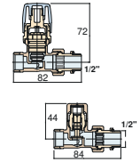
ПРЯМОЙ ВЕНТИЛЬ KRISTAL С ТЕРМОСТАТОМ, ХРОМИРОВАННЫЙ KRISTAL VALVE STRAIGHT WITH THERMOSTATIC OPTION CHROMED FINISHING
