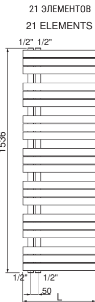
Центральное соединение (коллекторы слева) Detail of central connection (collectors on the right)
