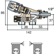
ДВУНАПРАВЛЕННЫЙ ВЕНТИЛЬ KRISTAL С БОКОВЫМ ВПУСКОМ И ТЕРМОСТАТОМ - БЕЛЫЙ R01 - RAL 9010 VALVE KRISTAL BIDIRECTIONAL LATERAL INLET WITH THERMOSTATIC OPTION - WHITE R01 - RAL 9010
