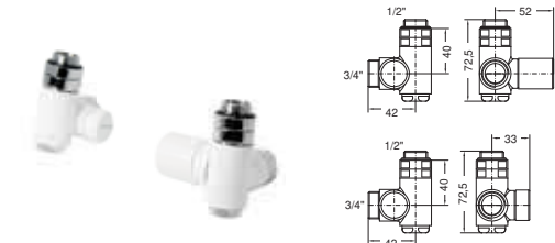
КОМБИНИРОВАННЫЙ ВЕНТИЛЬ KRISTAL С ТЕРМОСТАТОМ - БЕЛЫЙ R01 - RAL 9010 KRISTAL VALVE COMBI WITH THERMOSTATIC OPTION - WHITE R01 - RAL 9010
