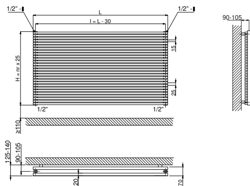
Размеры для клапанов типа Kristal Cordivari / Quotes for Kristal valves
