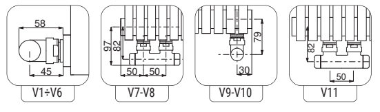
Размеры для клапанов типа Kristal Cordivari / Quotes for Kristal valves
