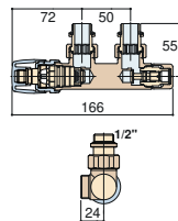
ЛЕВЫЙ ПРЯМОУГОЛЬНЫЙ ВЕНТИЛЬ KRISTAL, МЕЖСЕБЕВОЕ РАССТОЯНИЕ МЕЖДУ ТРУБАМИ 50 ММ, С ТЕРМОСТАТОМ - МАТОВАЯ ОТДЕЛКА KRISTAL VALVE SQUARE LEFT PIPE CENTRES 50 MM WITH THERMOSTATIC OPTION - SATIN FINISHING
