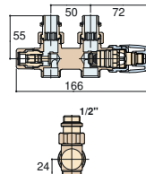
ПРЯМОЙ ВЕНТИЛЬ KRISTAL, МЕЖСЕБЕВОЕ РАССТОЯНИЕ МЕЖДУ ТРУБАМИ 50 ММ С ТЕРМОСТАТОМ - МАТОВАЯ ОТДЕЛКА KRISTAL VALVE STRAIGHT PIPE CENTRES 50 MM WITH THERMOSTATIC OPTION - SATIN FINISHING
