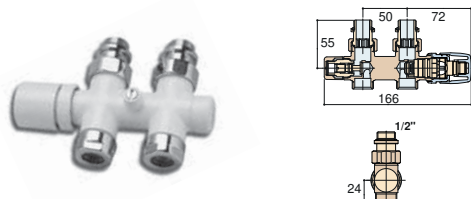
ПРАВЫЙ ПРЯМОЙ ВЕНТИЛЬ KRISTAL, МЕЖОСЕВОЕ РАССТОЯНИЕ МЕЖДУ ТРУБАМИ 50 MM, С ТЕРМОСТАТОМ - БЕЛЫЙ R01 - RAL 9010 KRISTAL VALVE STRAIGHT RIGHT PIPE CENTRES 50 MM WITH THERMOSTATIC OPTION - WHITE R01 - RAL 9010
